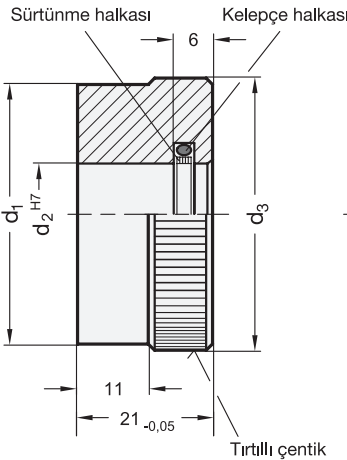
Sürtünme halkalı versiyon için bağlantı ölçüleri
