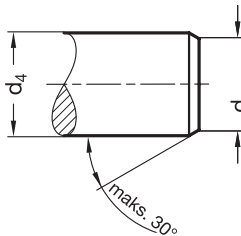
Sürtünme halkalı versiyon için bağlantı ölçüleri
